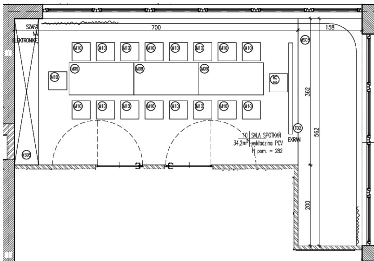
Schemat nr 1 – rzut Sali Wielofunkcyjnej
